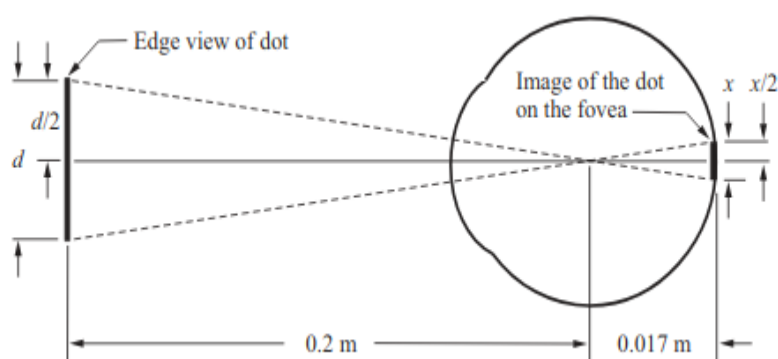
Figura 2: Esquema geral. O ponto de diâmetro " d " mm se projetando sobre um sensor de " x " mm.
